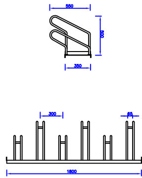
APARCAMIENTO DE BICIS
