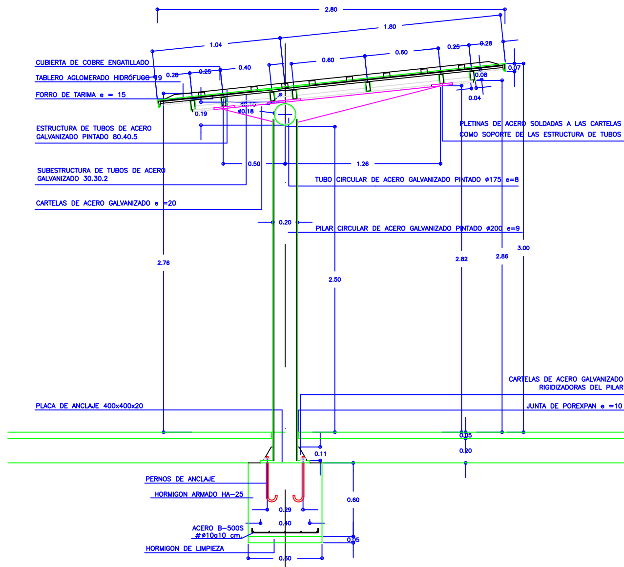
SECCION A - A
