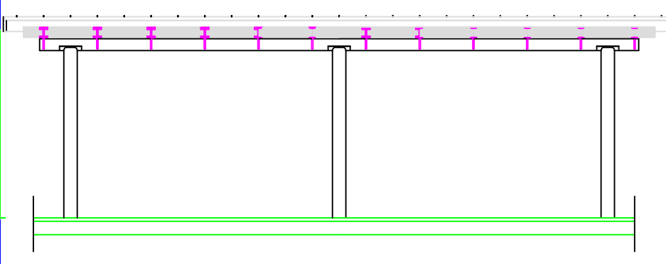
ALZADO FRONTAL E : 1/80
