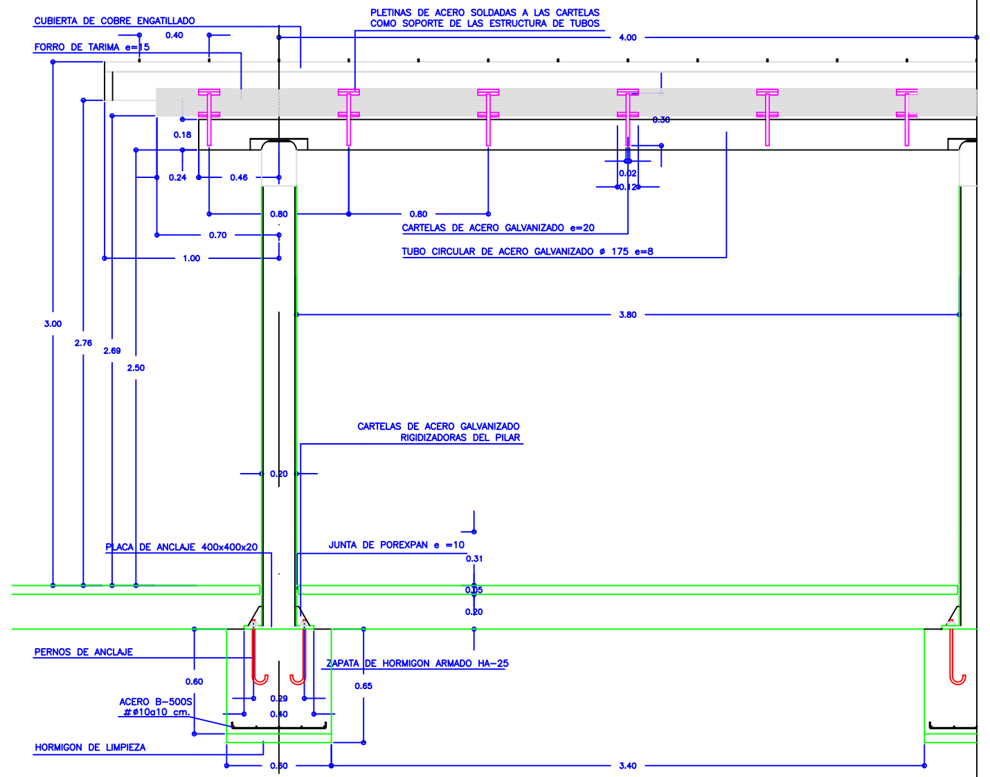
SECCION B - B
