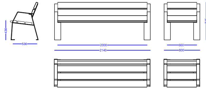
BANCO Y SILLA
