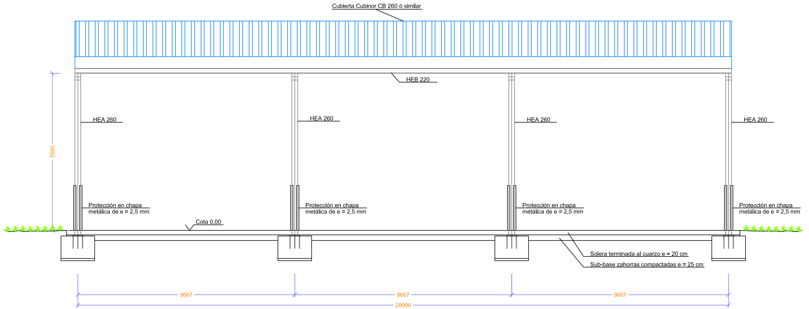
ALZADO LATERAL
